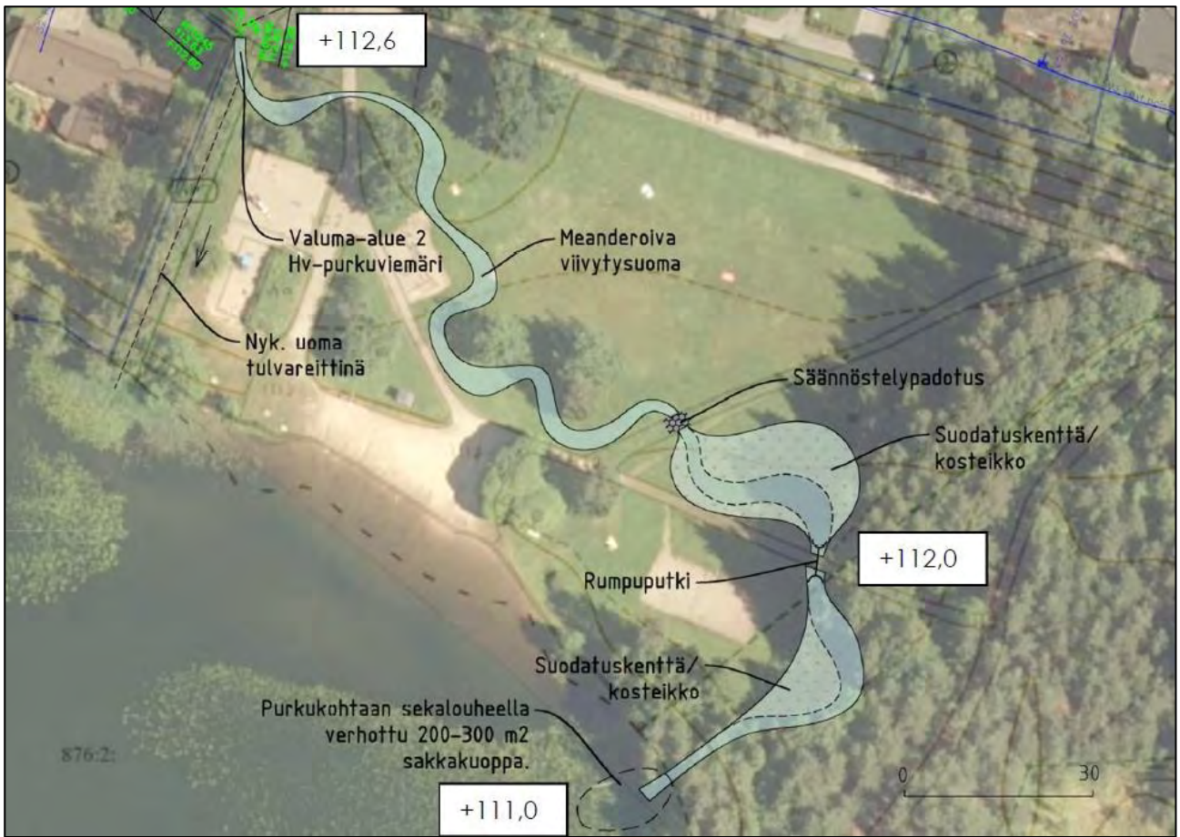
Kuva 8. Ideokuva Suopursunpuiston hulevesien viivytyksestä (WSP).
