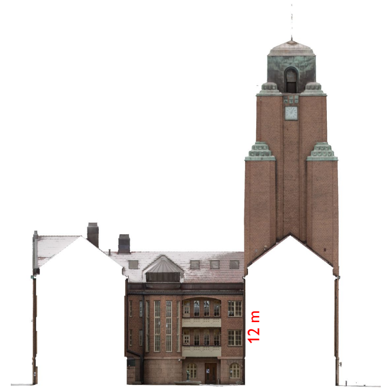
Julkisivu itään
