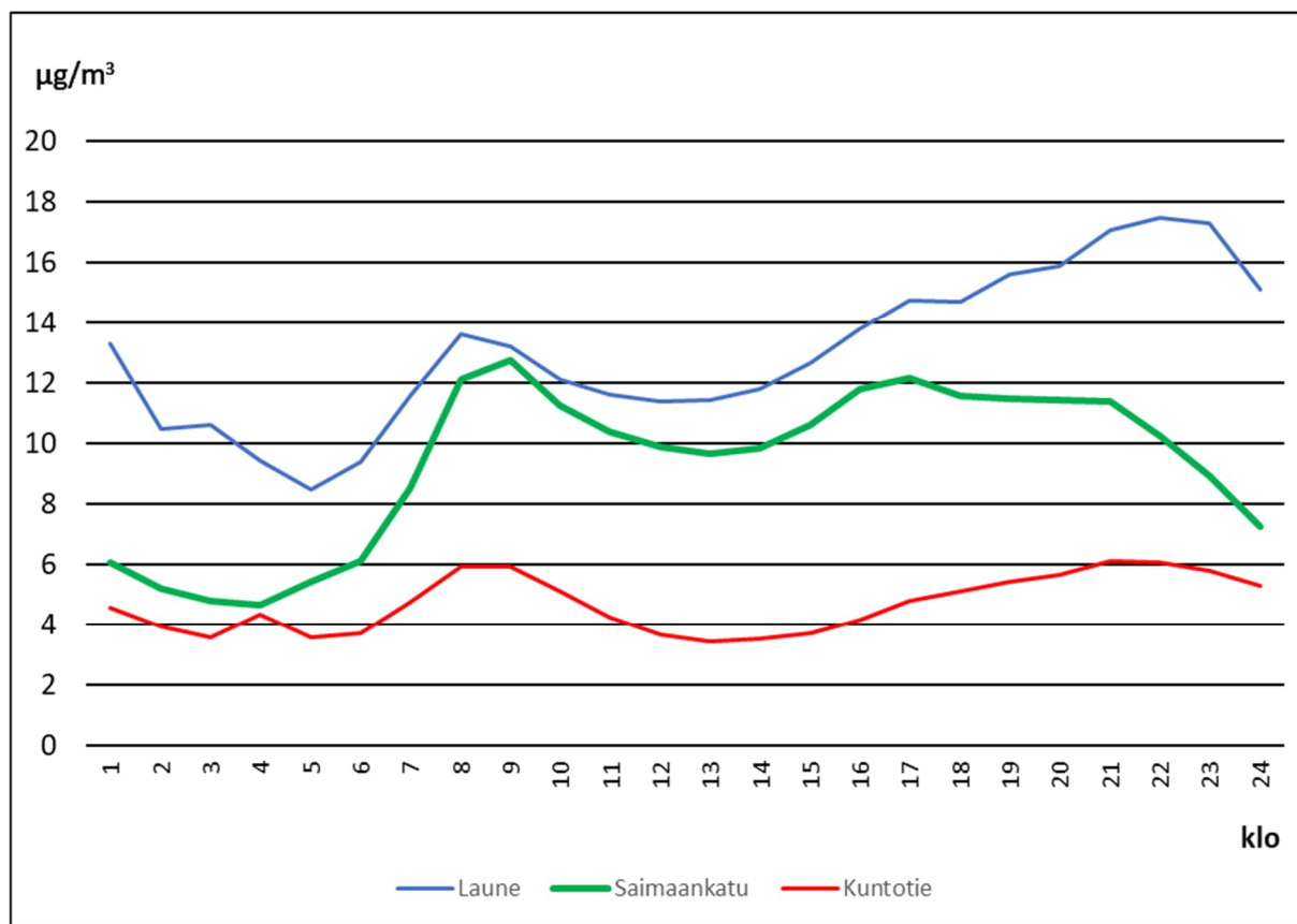
Kuva 12. Typpidioksidipitoisuuksien tuntikeskiarvot tunneittain Lahden seudulla vuonna 2023.
