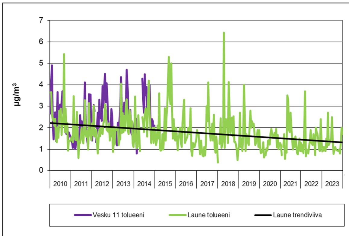
Kuva 27. Tolueneipitoisuudet Launeella vuosina 2010–2023 ja Vesku 11 mittauspisteessä vuosina 2010–2014. (Vesku 11 mittauspisteessä mittaukset lopetettiin vuonna 2014).
