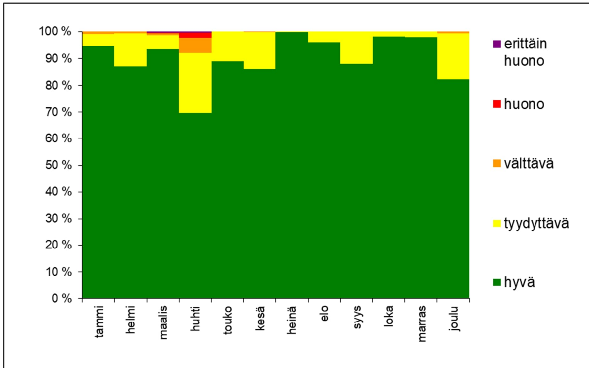
Kuva 37. Ilmanlaatuindeksit vuonna 2023 Kuntotien mittausasemalla.
