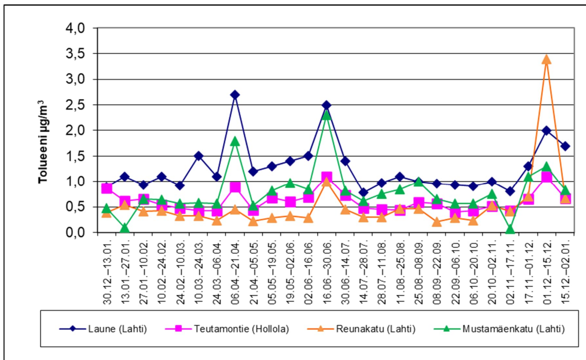
Kuva 28. Tolueneipitoisuudet Lahden seudulla vuonna 2023.
