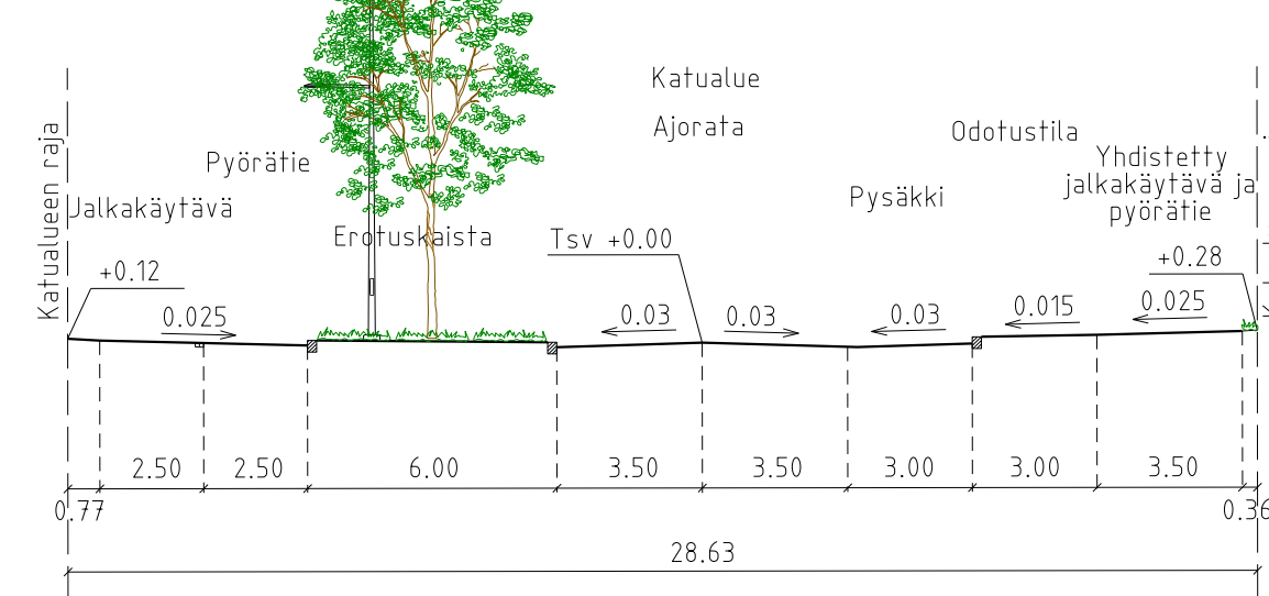
POIKKILEIKKAUS B - B 1:200
