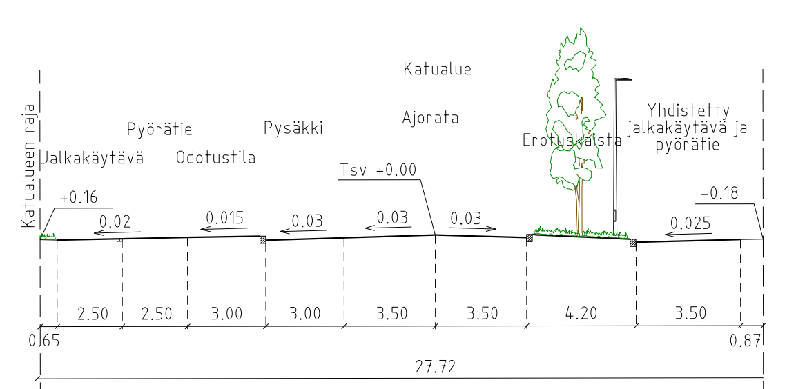
POIKKILEIKKAUS D - D 1:200
