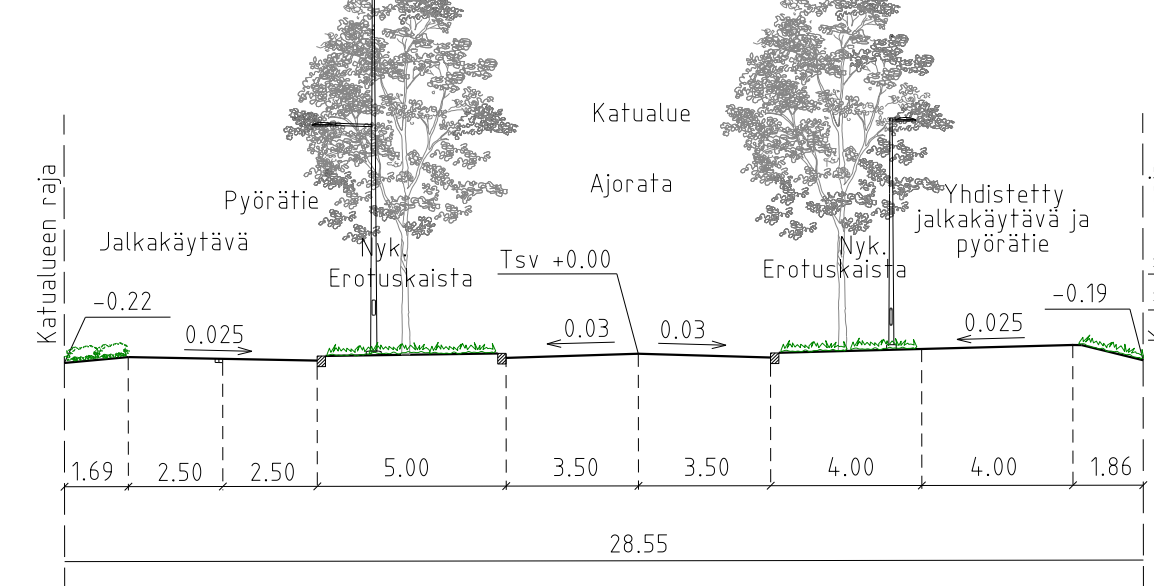
POIKKILEIKKAUS C - C 1:200
