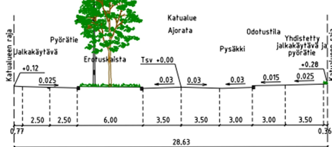
POIKKILEIKKAUS B - B 1:200
