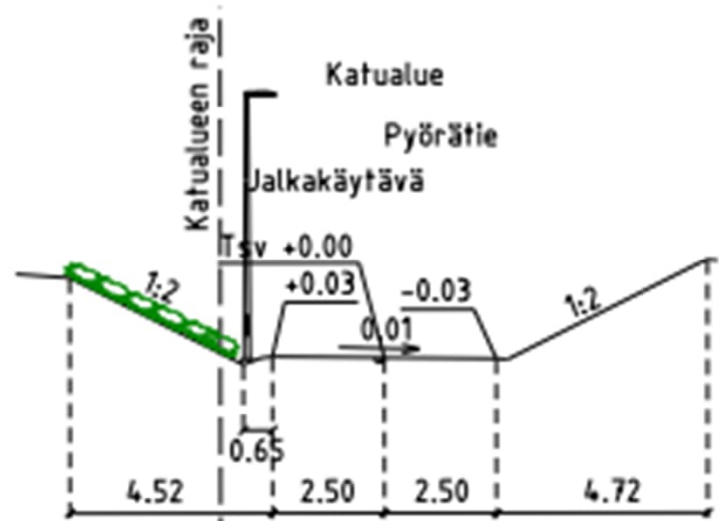
POIKKILEIKKAUS A - A 1:200
