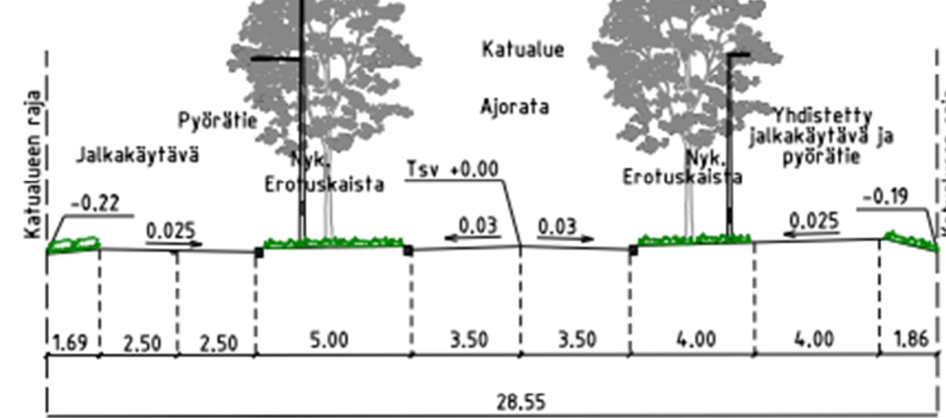
POIKKILEIKKAUS C - C 1:200
